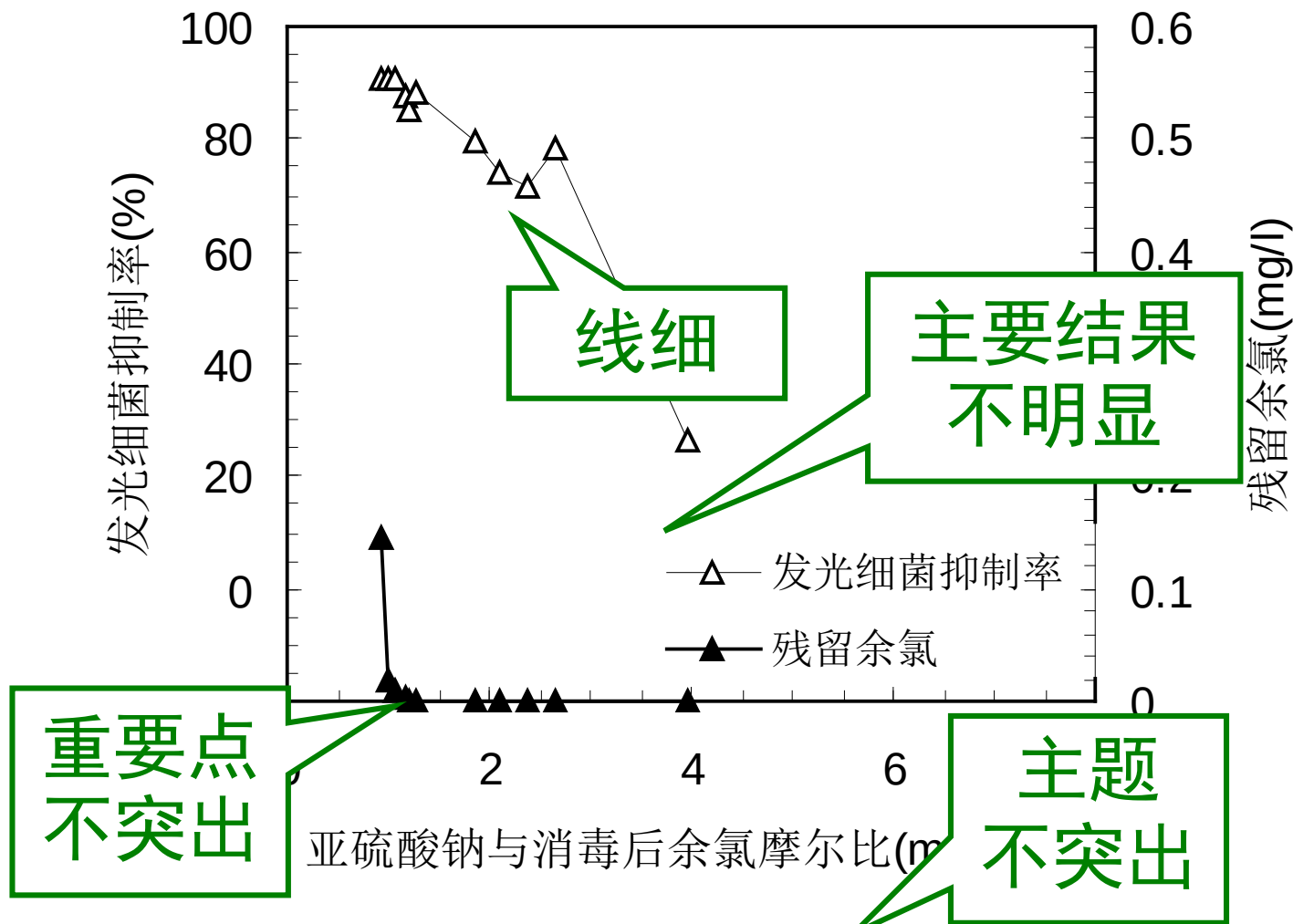
图2.4 某厂出水消毒后的生物毒性随硫氯比的变化
