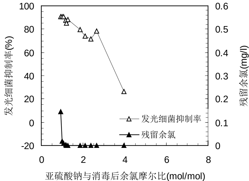
图2.4 某厂出水消毒后的生物毒性随硫氯比的变化
